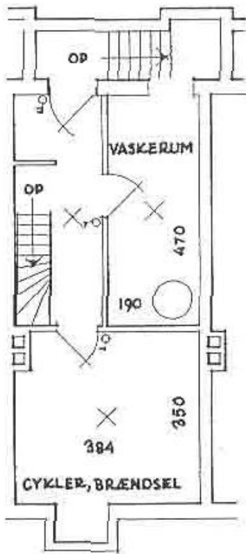
Kælderplan
